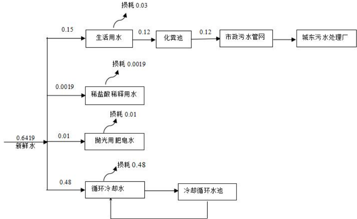
建设项目水平衡图 (t/d)
