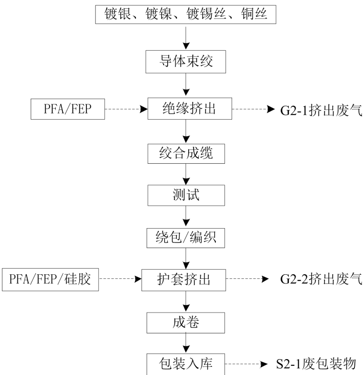
图 2-2 航空航天专用线缆生产工艺流程及产污环节图
