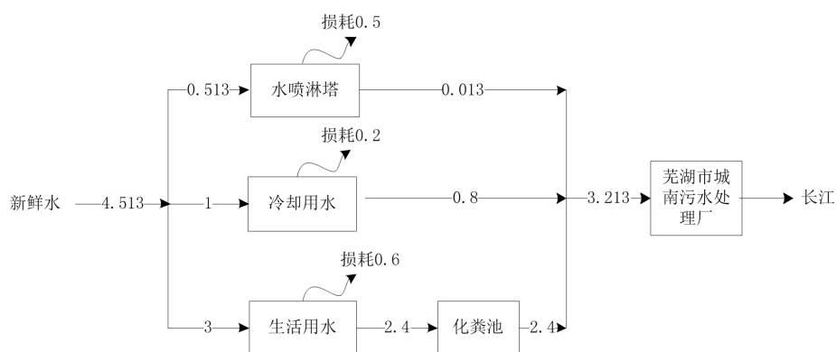
图 4-2 项目水平衡图 (单位: t/d)
