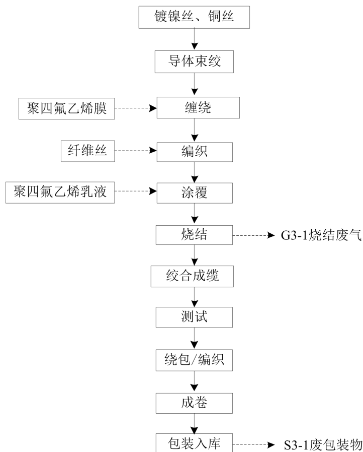
图 2-3 舰船专用线缆生产工艺流程及产污环节图
